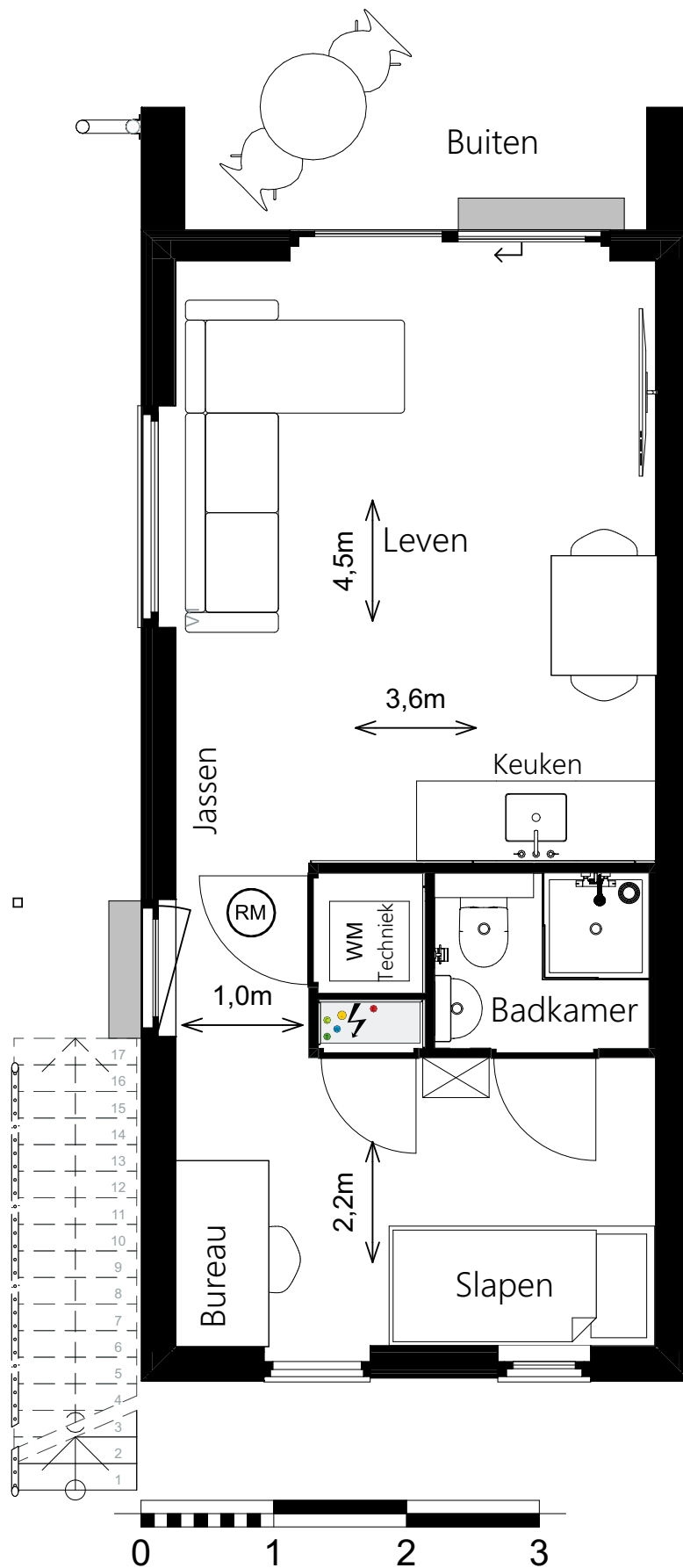
Begane grond - Éénpersoonswoning gestapeld
