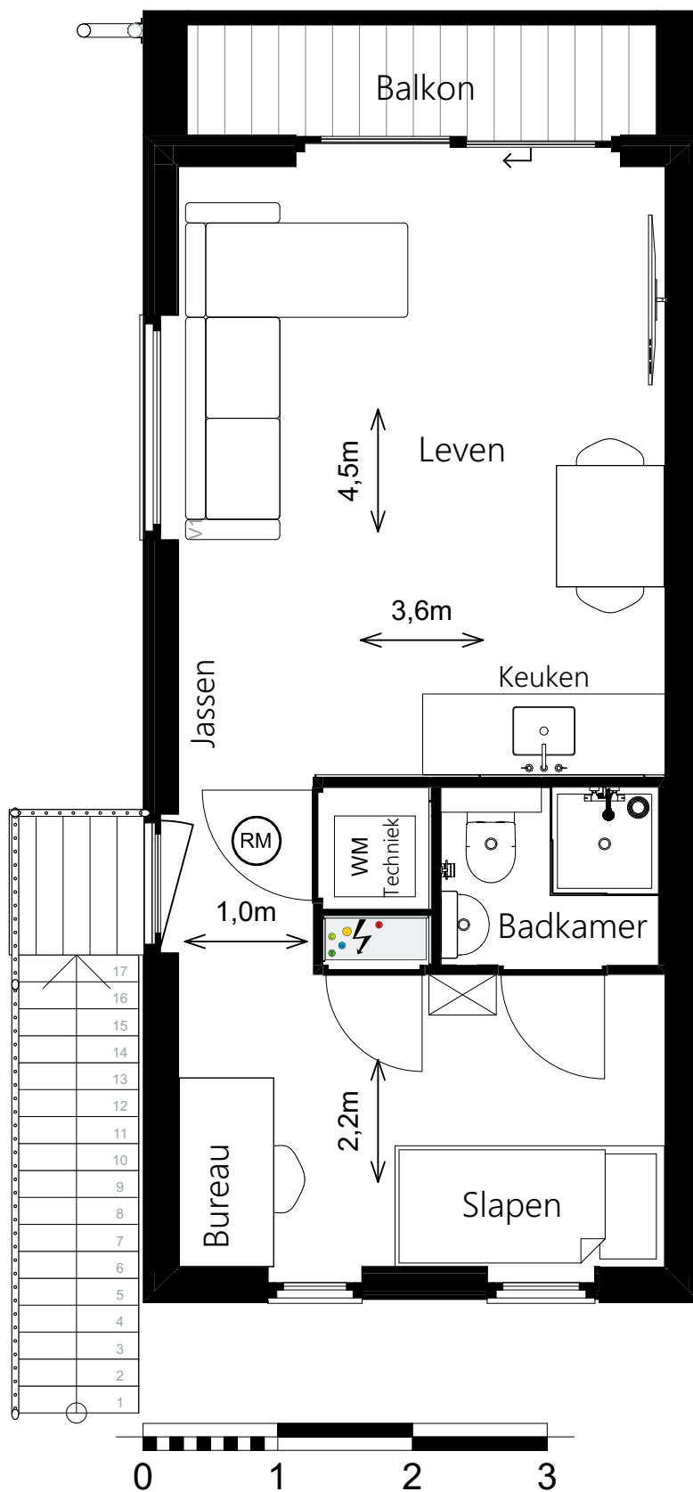
1e verdieping - Éénpersoonswoning gestapeld
