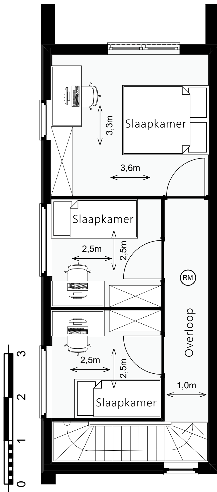
1e verdieping - Gezinswoning
