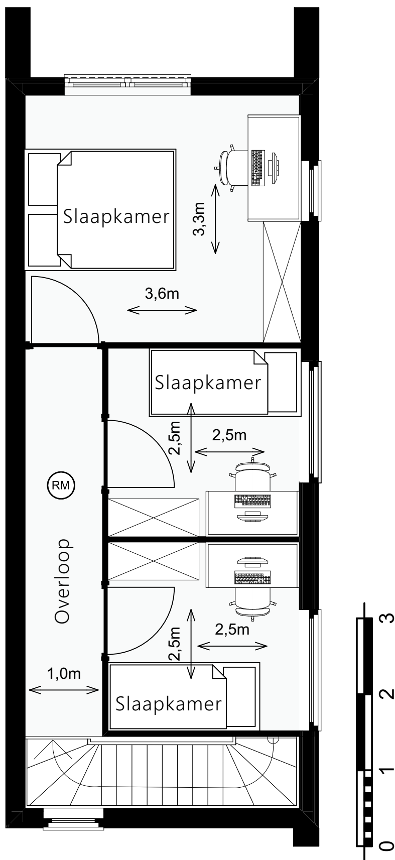
1e verdieping gespiegeld - Gezinswoning
