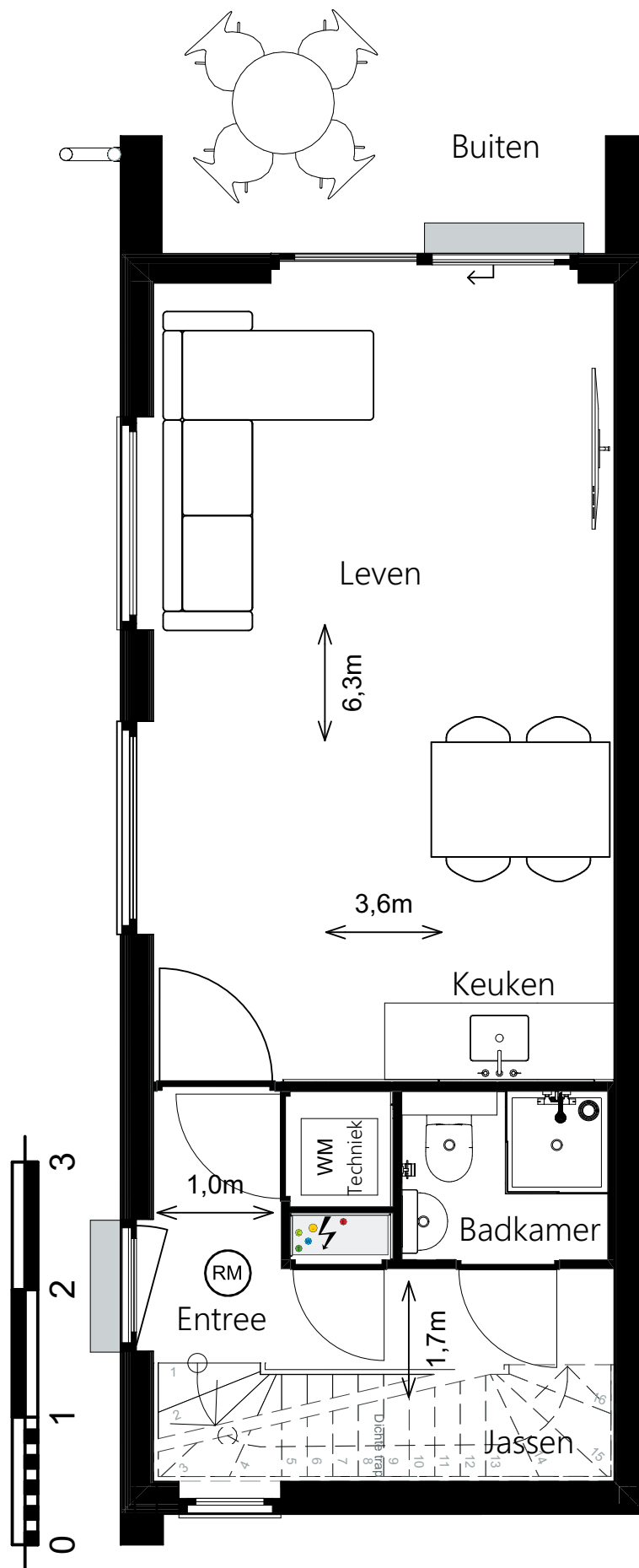
Begane grond - Gezinswoning
