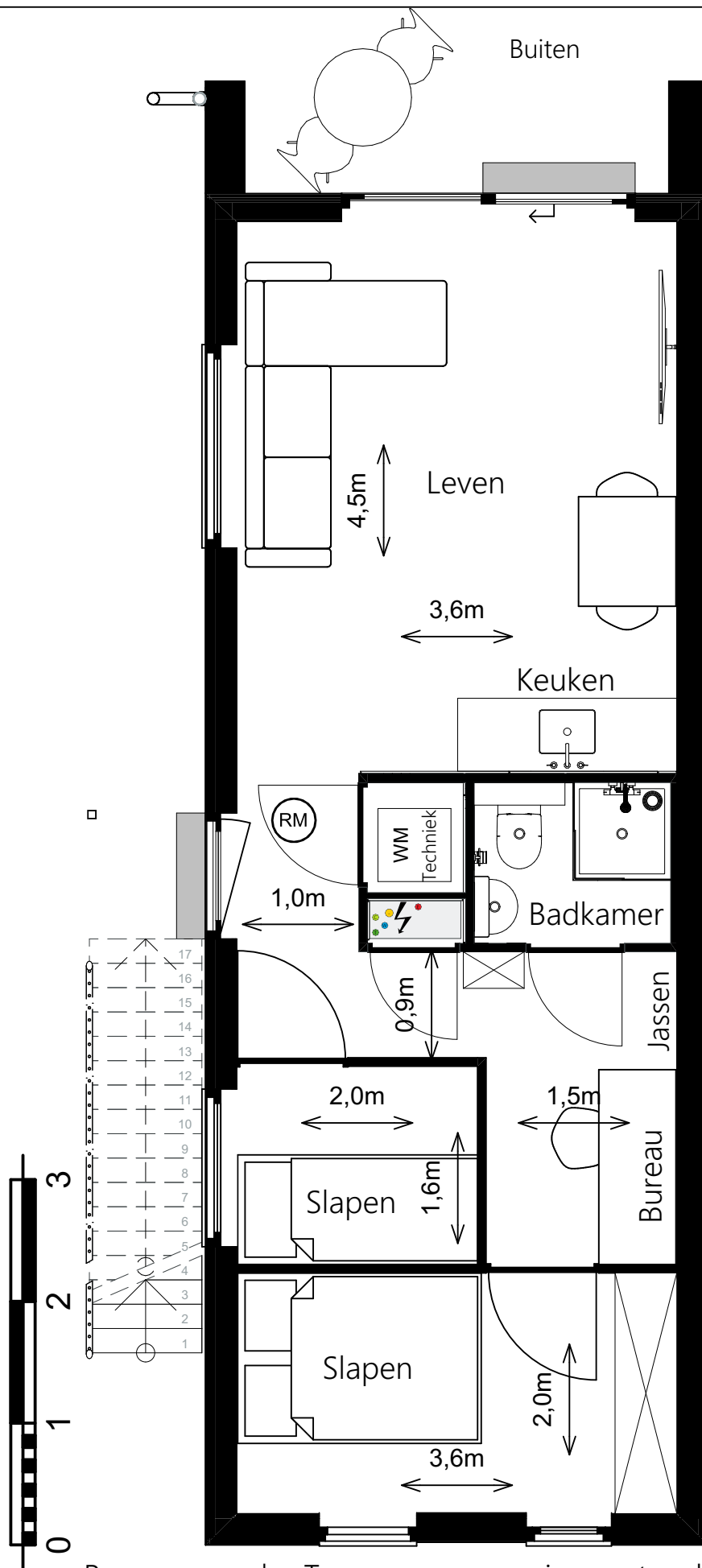
Begane grond - Tweepersoonswoning gestapeld
